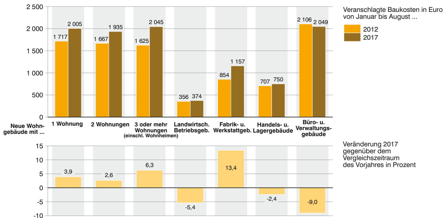
Abb. 6 Veranschlagte Baukosten je m 2 Wohn- bzw. Nutzfläche im Neubau in Bayern von Januar bis August 2012 und 2017
